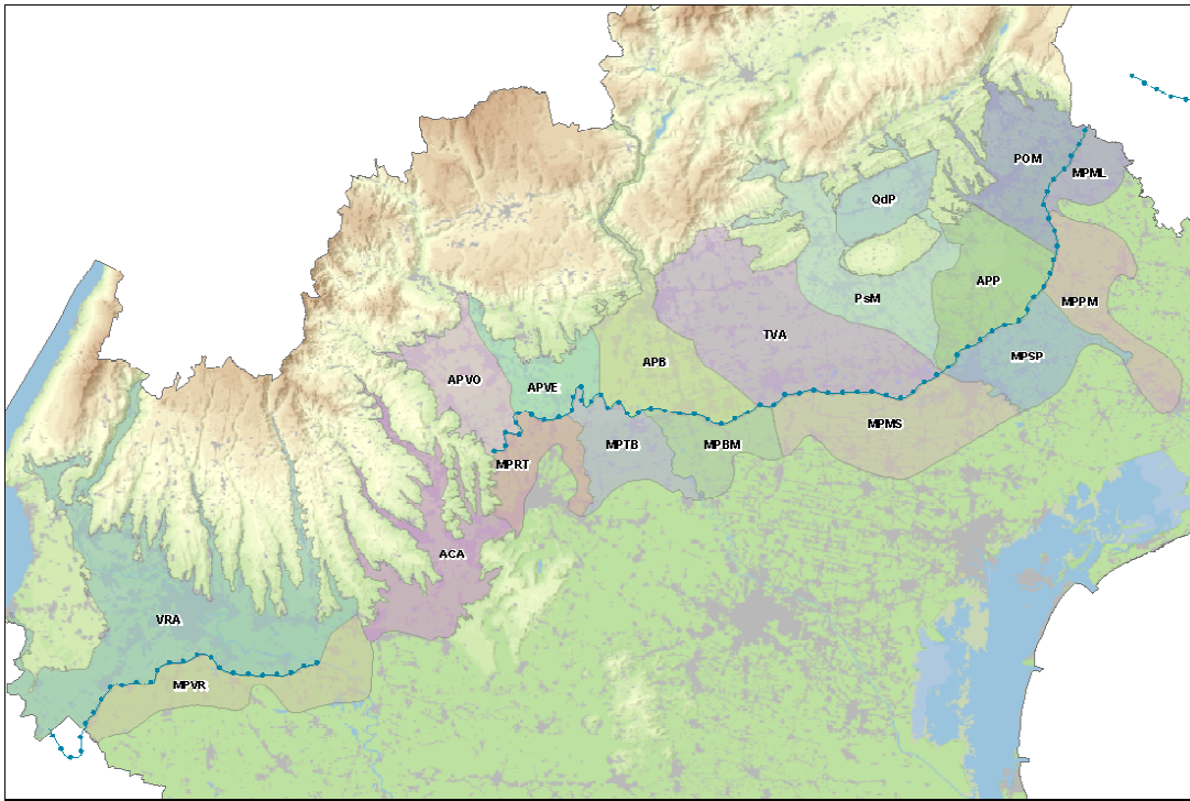
Figura A.13: bacini Idrogeologici della Pianura Veneta.
