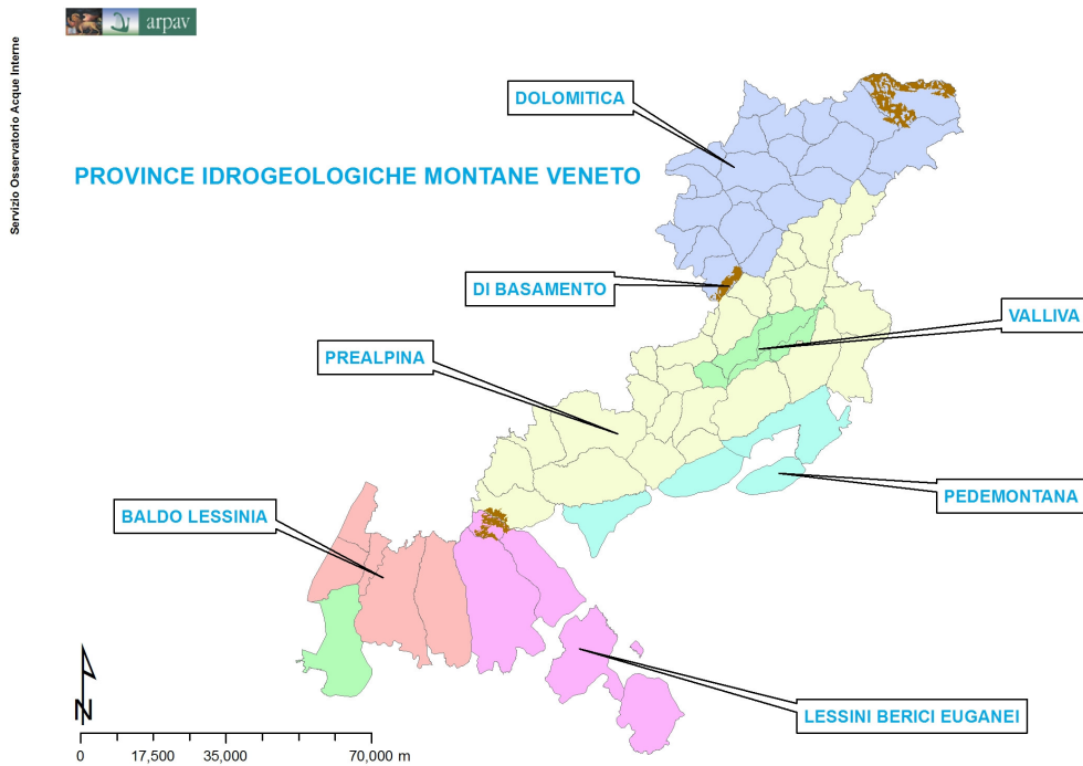
Figura A.14: province idrogeologiche della zona montana Veneta.
