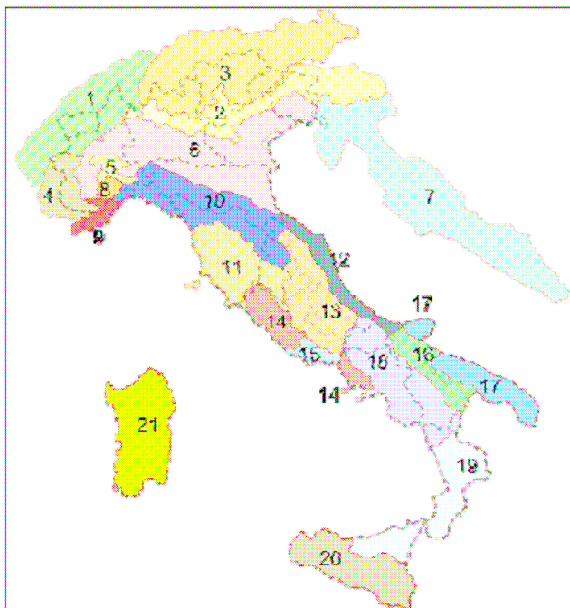
Figura A.1: idro-ecoregioni individuate dal CEMAGREF che interessano l'Italia.
