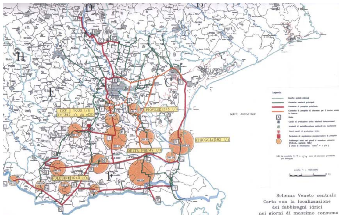
Figura 2.15 - Reti di interconnessione e localizzazione dei fabbisogni idrici
