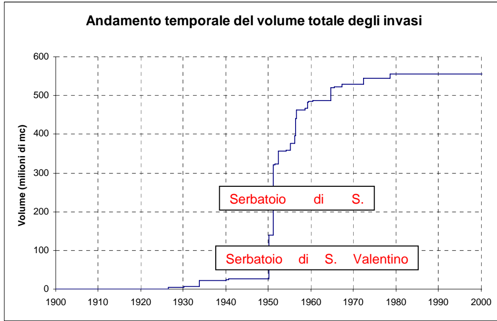
Figura 2.17 - Variazione temporale del volume invasabile dai serbatoi artificiali.
