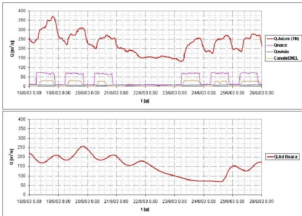
Figura 2.19 - Andamento tipico delle portate a Trento e Boara Pisani in periodo estivo
