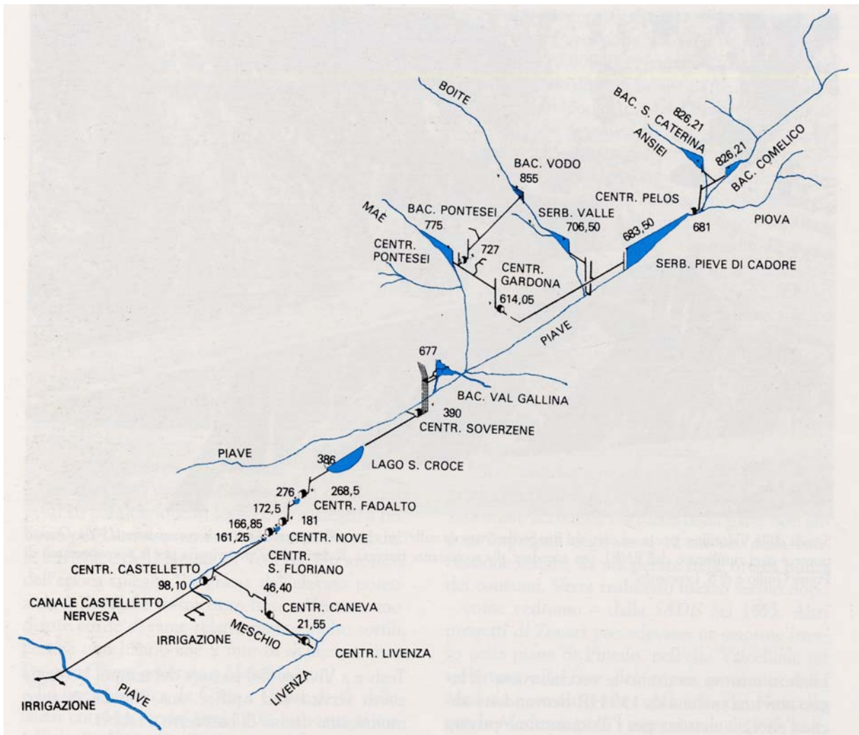
Figura 2.20: Schema del collegamento delle acque del Piave – Santa Croce – Livenza.
