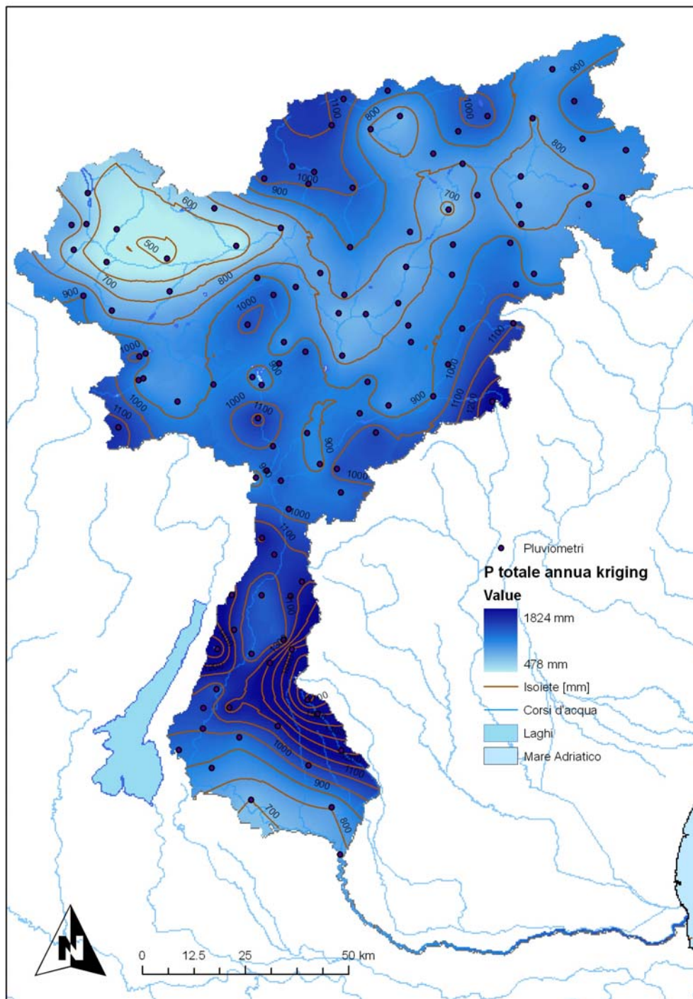
Figura I4 -Precipitazione media nel bacino dell'Adige.
