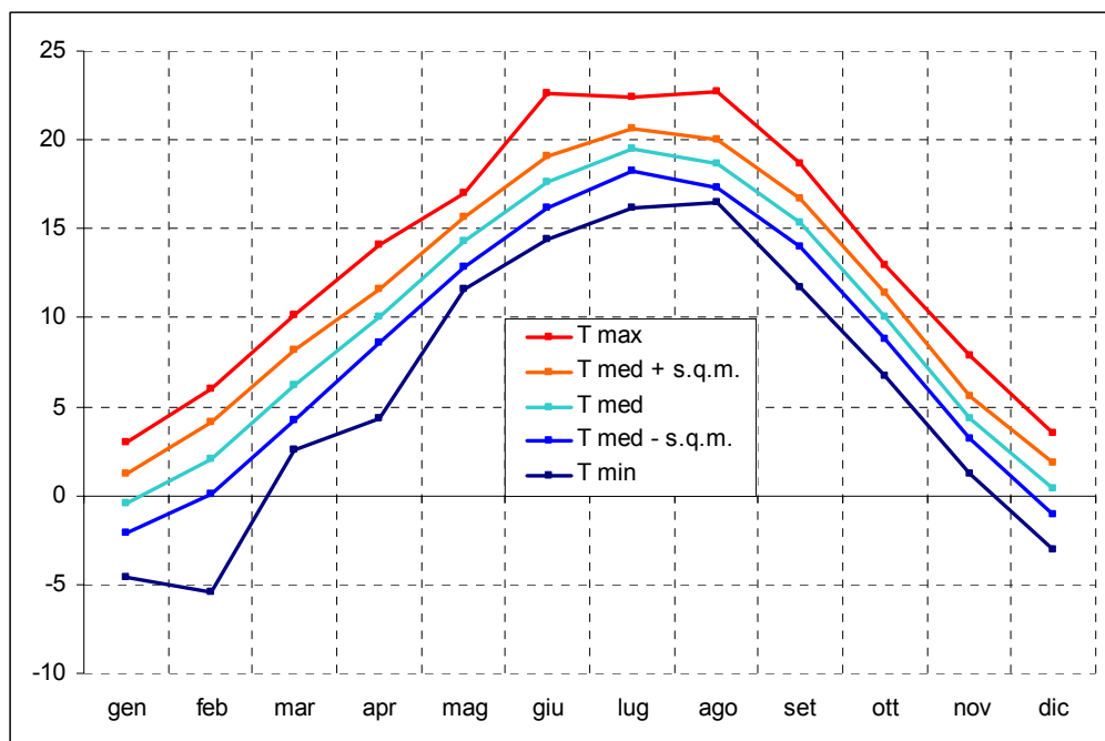
Figura 17 - Stazione di Silandro – Regime medio della temperatura
