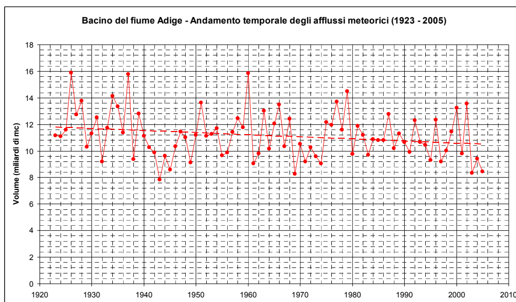
Figura I5 - Andamento temporale degli afflussi meteorici
