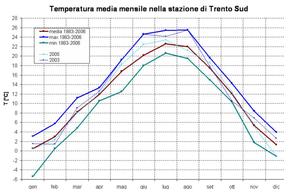
Figura I6 - Andamento della temperatura media mensile nella stazione di Trento Sud.
