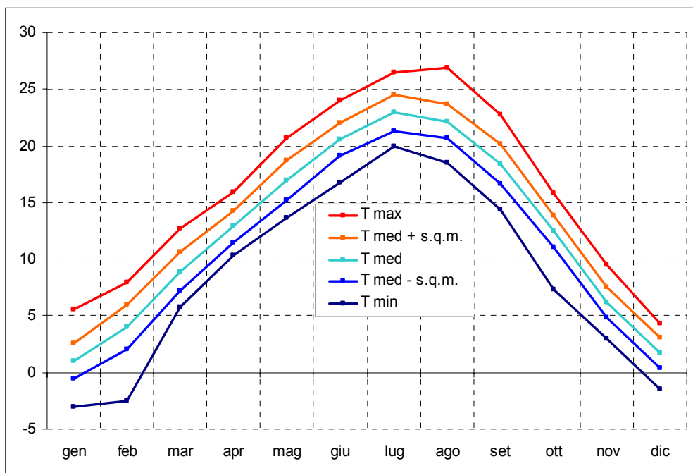
Figura I8 - -Stazione di Trento Laste – Regime medio della temperatura
