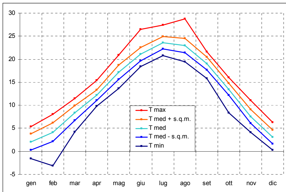
Figura I9 - Stazione di Villafranca Veronese – Regime medio della temperatura
