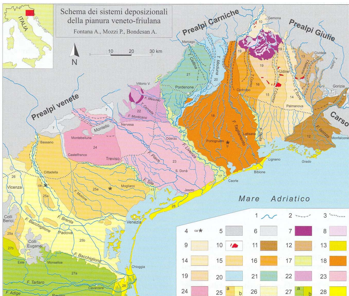
Figura I. 9: schema dei sistemi deposizionali della pianura veneto-friulana (Fonte: "Geomorfologia della Provincia di Venezia", AA.VV., Prov. VE, 2004).
