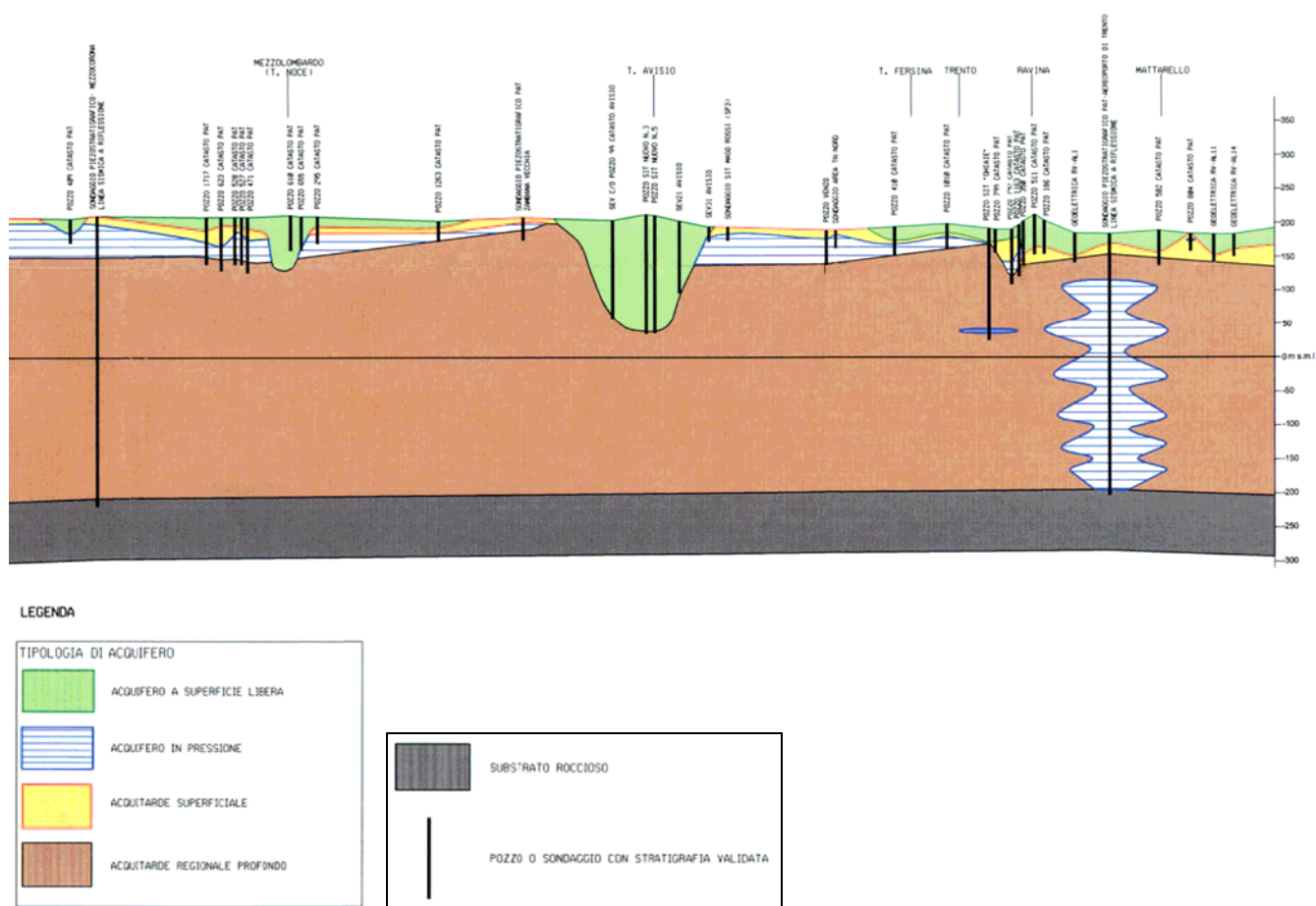
Figura I. 14: profilo idrogeologico schematico del fondovalle atesino.
