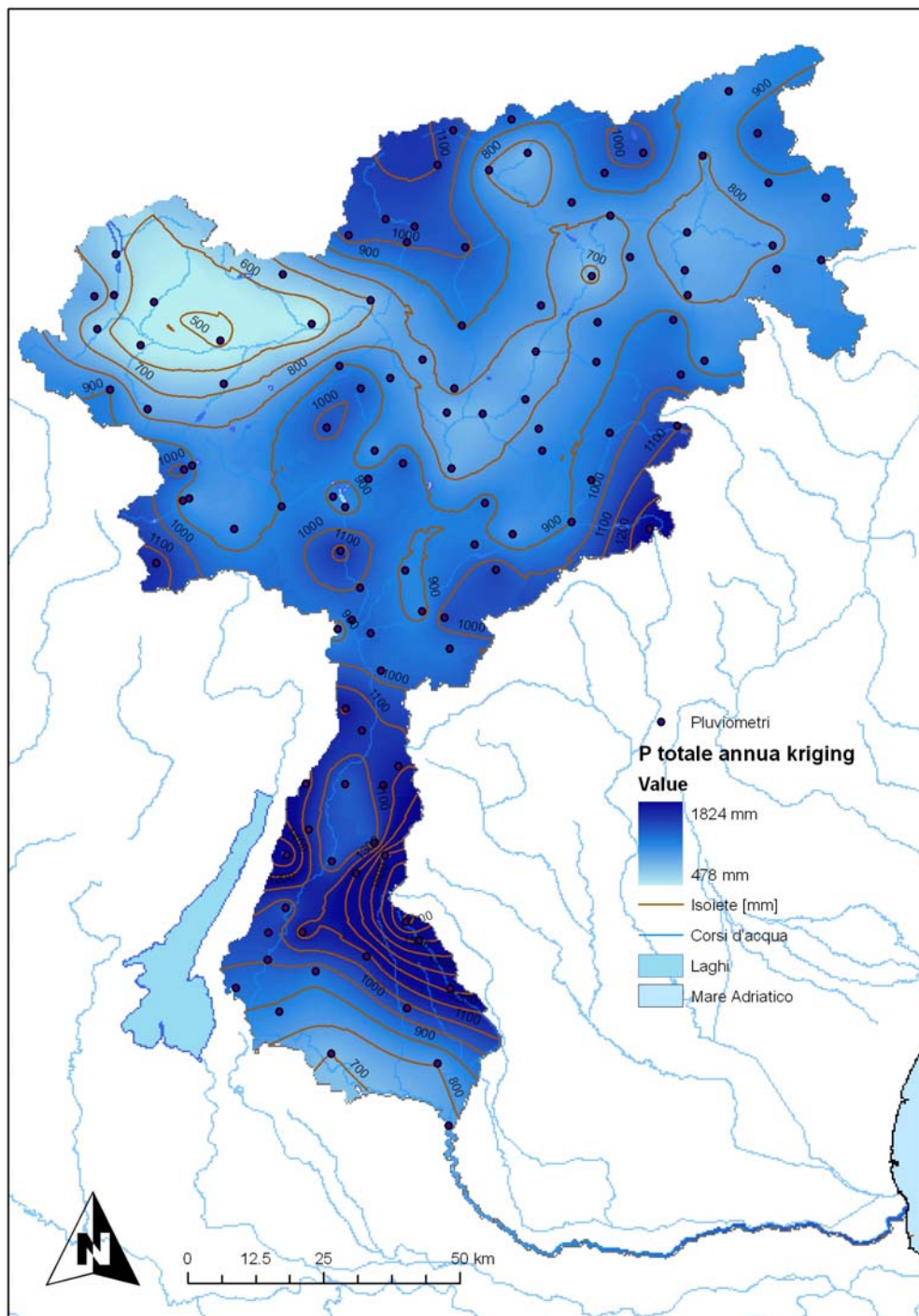
Figura I. 3: precipitazione media annua nel bacino dell'Adige.
