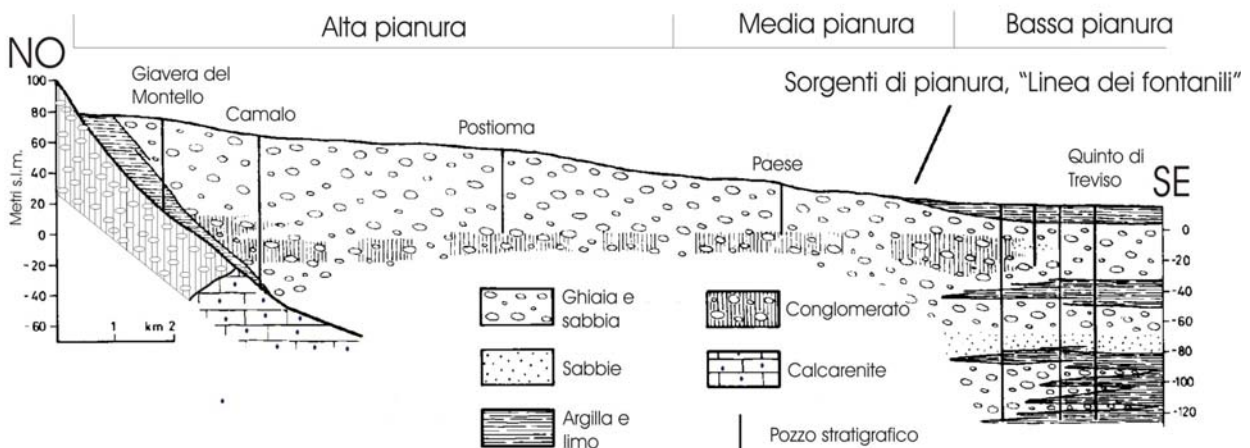
Figura I. 11: sezione geologica schematica trasversale alla Pianura Veneta, con andamento NO – SE. (Fonte: Vorliceck, Antonelli, Fabbri, Rausch. "Quantitative hydrogeological studies of Treviso alluvial plain (NE Italy)", in stampa nel Quarterly Journal of engineering geology and hydrogeology della Geological Society of London).
