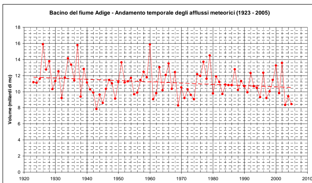
Figura I. 4: andamento temporale degli afflussi meteorici.
