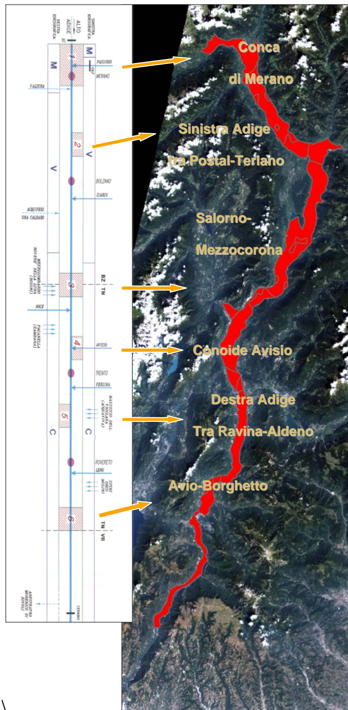
Figura I. 13: carta tematica di sintesi sull'ubicazione e caratteri idrogeologici dell'acquifero alluvionale di fondovalle dell'Adige.
