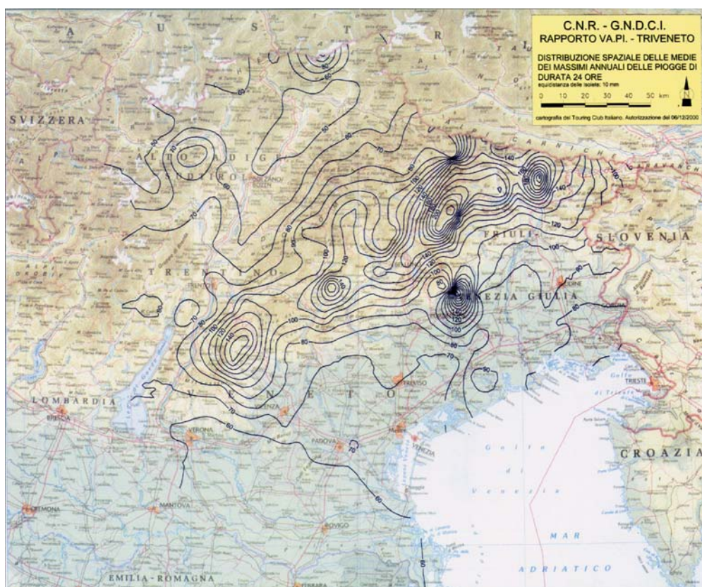
Figura 12: carta isoietografica riferita alla media dei massimi annuali di pioggia di durata di 24 ore.
