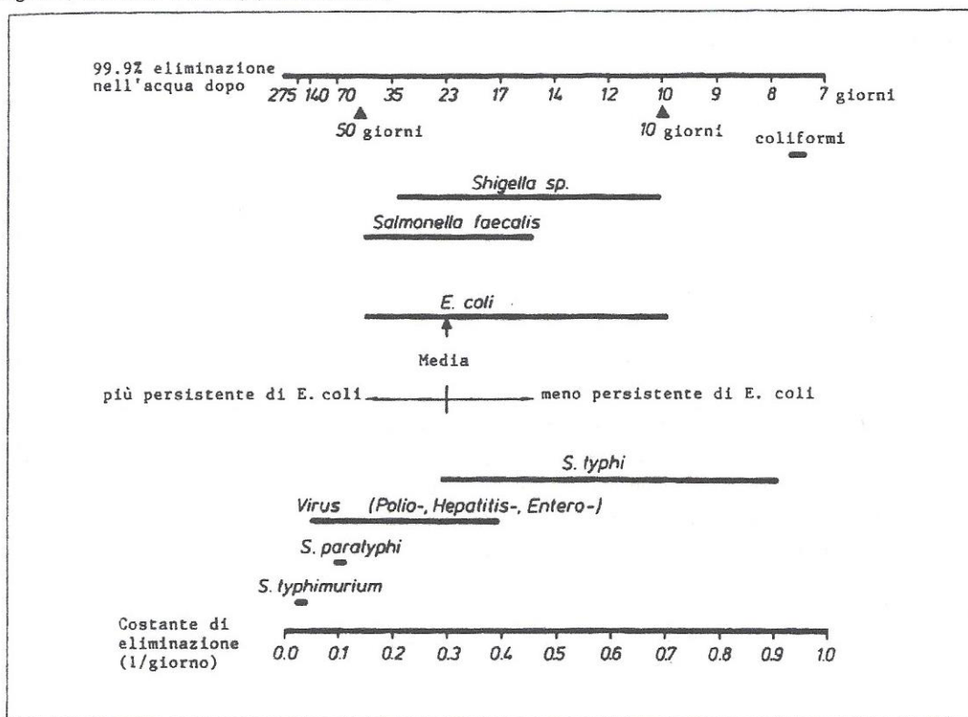
Figura 1 – Costante di eliminazione (l/giorno) ed eliminazione al 99,9% di batteri e virus presenti nelle acque sotterranee (Pekdeger A., Mattheess G., 1982) (da Beretta1992)
